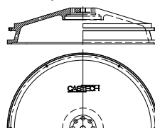
Lemiesz I rys. nr 15-4C2
